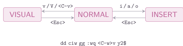
Figure 6: El mapa de teclado modal de Vim y su notación viajera. Los modos (NORMAL, INSERT, VISUAL) están conectados por transiciones de pulsaciones etiquetadas; los comandos comunes ( dd borrar-línea, ciw cambiar-palabra-interna, gg ir-arriba, :wq escribir-y-salir, etc.) son la moneda discursiva del mapa de teclado. La notación es tan portátil que se ha reimplementado en VS Code, JupyterLab, Vimium, el sistema de texto Cocoa de macOS y set -o vi .
