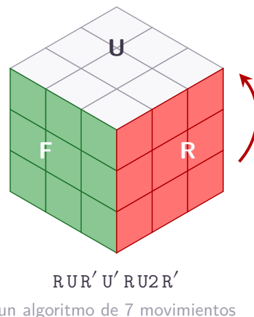
Figure 7: La notación de cubo de Singmaster [Singmaster, 1981]. Cada letra mayúscula nombra una cara (Up/arriba, Down/abajo, Left/izquierda, Right/derecha, Front/frente, Back/atrás); una letra sola es un cuarto de giro horario, una letra con prima (') un cuarto de giro antihorario, y un dígito 2 un medio giro. La cadena de siete símbolos R U R' U' R U2 R' es un algoritmo completo portátil entre cuberos, repositorios de GitHub y tutoriales de YouTube — el par mapa de teclado-notación viajando como texto. Las caras llevan el esquema de pegatinas estándar (blanco arriba, verde al frente, rojo a la derecha); R está dibujada a medio cuarto de giro: el primer movimiento del algoritmo.
