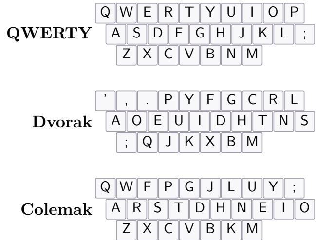
Figure 2: Tres mapas de teclado de escritura sobre el mismo sustrato físico. Cada diseño es una reasignación de posiciones de teclas idénticas a un conjunto distinto de letras. QWERTY (Sholes 1873, nunca patentado), Dvorak (Dvorak & Dealey 1936, US 2,040,248), Colemak (Coleman 2006, dominio público). El ecosistema de bifurcaciones posterior a 2010 prolonga esta línea.
