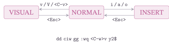
Figure 6: Модальная раскладка Vim и её путешествующая нотация. Режимы (NORMAL, INSERT, VISUAL) соединены помеченными переходами по нажатиям; распространённые команды ( dd удалить строку, ciw изменить внутреннее слово, gg к началу, :wq записать и выйти и т.д.) — дискурсивная валюта раскладки. Нотация столь переносима, что перереализована в VS Code, JupyterLab, Vimium, текстовой системе macOS Cocoa и set -o vi .
