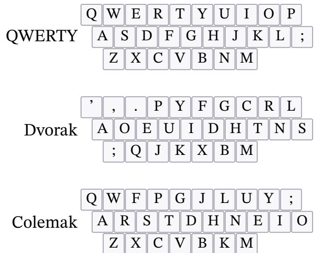
Figure 2: Три печатные раскладки над одним физическим субстратом. Каждая раскладка — это перепривязка одних и тех же позиций клавиш к иному набору букв. QWERTY (Шоулз 1873, никогда не патентовалась), Dvorak (Dvorak и Dealey 1936, US 2,040,248), Colemak (Coleman 2006, общественное достояние). Экосистема форков после 2010 года продолжает эту линию.
