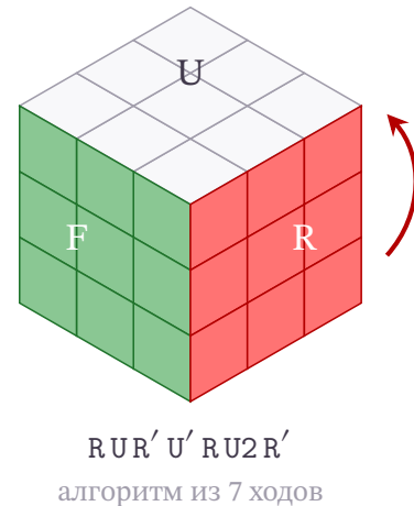
Figure 7: Кубическая нотация Сингмастера [Singmaster, 1981]. Каждая заглавная буква именуется грань (Up — верх, Down — низ, Left — лево, Right — право, Front — перед, Back — зад); голая буква — поворот на четверть по часовой стрелке, штрихованная буква (') — против часовой, а цифра-2 — полуоборот. Строка из семи токенов RUR' U' RU2R'' — полный алгоритм, переносимый между куберами, репозиториями GitHub и видеороликами YouTube, — пара раскладкано-нотация, путешествующая как текст. Грани несут стандартную схему наклеек (белый — верх, зелёный — перед, красный — право); R нарисована в середине четвертьповорота: первый ход алгоритма.
