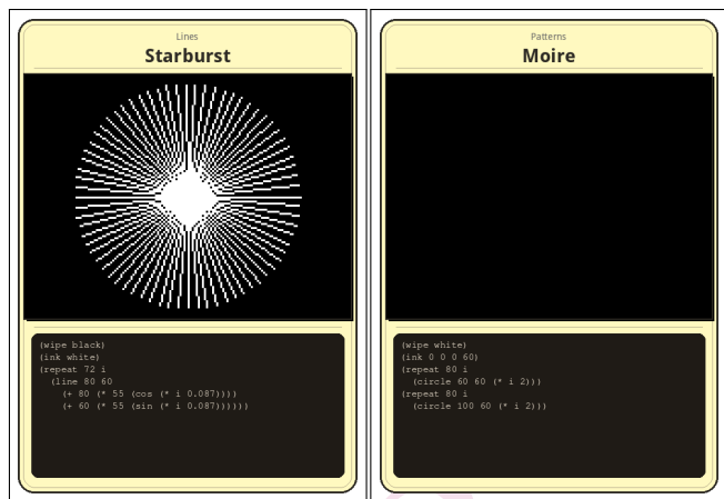
Figure 1: Dos tarjetas de programa renderizadas por el intérprete Python: “Starburst” (72 líneas radiales, 3 líneas de código) y “Moiré” (círculos concéntricos superpuestos, 3 líneas). Estos son ejemplos triviales—demuestran la estructura del formato pero no representan el rango expresivo del lenguaje ni las ambiciones del formato.
