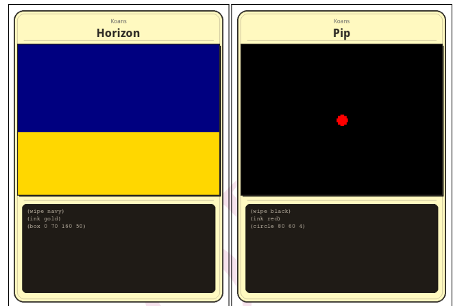
Figure 6: “Horizon” y “Pip” — koans mínimos (2–3 líneas cada uno).
