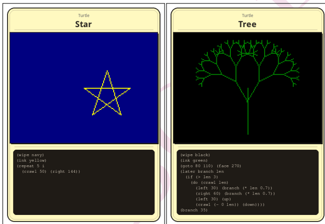
Figure 5: “Star” y “Tree” — tarjetas de gráficos de tortuga.
