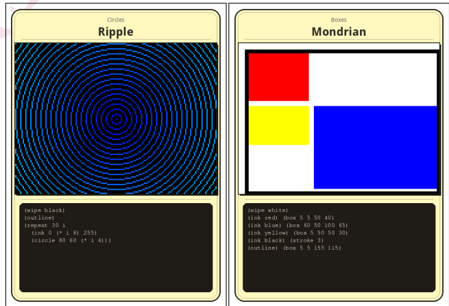
Figure 3: “Ripple” (círculos) y “Mondrian” (cajas).
