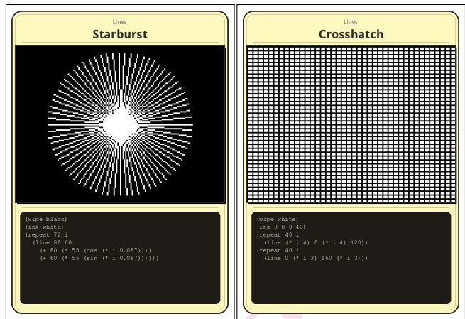
Figure 2: “Starburst” y “Crosshatch” — tarjetas de líneas.
