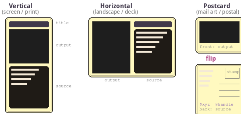
Figure 8: Tres estrategias de disposición. Vertical: título / imagen / fuente apilados de arriba a abajo, optimizado para pantallas de teléfono e impresión en retrato. Horizontal: imagen a la izquierda, título y fuente a la derecha, adecuado para tarjetas en paisaje y navegación de baraja lado a lado. Postal: salida renderizada en el frente, código fuente y metadatos en el reverso—una tarjeta enviable por correo donde el programa está oculto hasta que la volteas.
