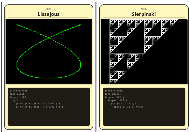
Figure 4: “Lissajous” (curvas matemáticas) y “Sierpinski” (fractal AND a nivel de bits).
