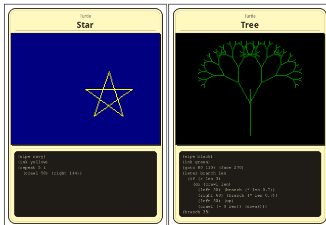
Figure 5: “Star” 和 “Tree” — 海龟图形卡片。
