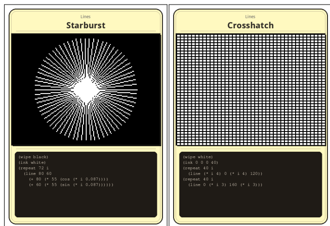
Figure 2: “Starburst” 和 “Crosshatch” — 线条卡片。
