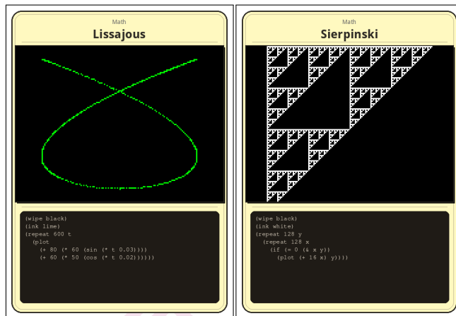
Figure 4: “Lissajous” (数学曲线) 和 “Sierpinski” (位与分形)。
