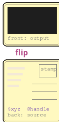
Figure 8: 三种布局策略。纵向：标题/图像/源代码从上到下堆叠，针对手机屏幕和纵向打印优化。横向：图像在左，标题和源代码在右，适合横向卡片和并排浏览。明信片：正面是渲染输出，背面是源代码和元数据——一张可邮寄的卡片，翻转后才能看到程序。
