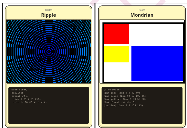
Figure 3: “Ripple” (圆形) 和 “Mondrian” (方块)。
