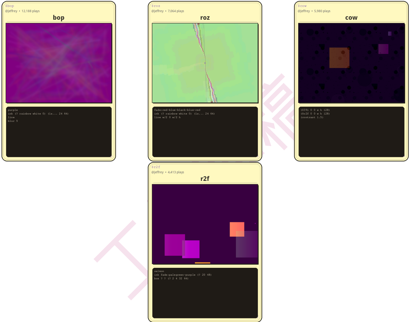
Figure 11: 来自 KidLisp 活跃语料库的四张卡片，由 oven 服务渲染。从左到右：$bop (12,188 次播放——最受欢迎的作品，4 行)，$roz (7,064 次播放，3 行)，$cow (5,980 次播放——通过 $39i 和 $r2f 嵌入其他两个作品的组合)，$r2f (4,413 次播放，3 行随机方块放置)。全部出自 @jeffrey。这些程序使用了 Python 解释器中不存在的功能——动画、随机性 (?)、渐变淡出 (fade:)、嵌入层 ($code)——但它们的源代码仍然放得下一张卡片。
